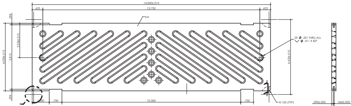
DETAIL: SVI-4x14-B
