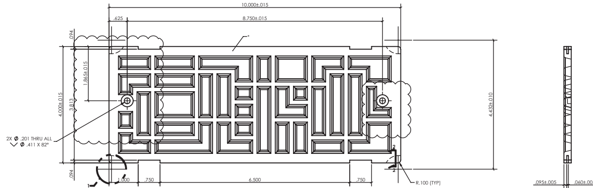
DETAIL: SVI-4x10-T
