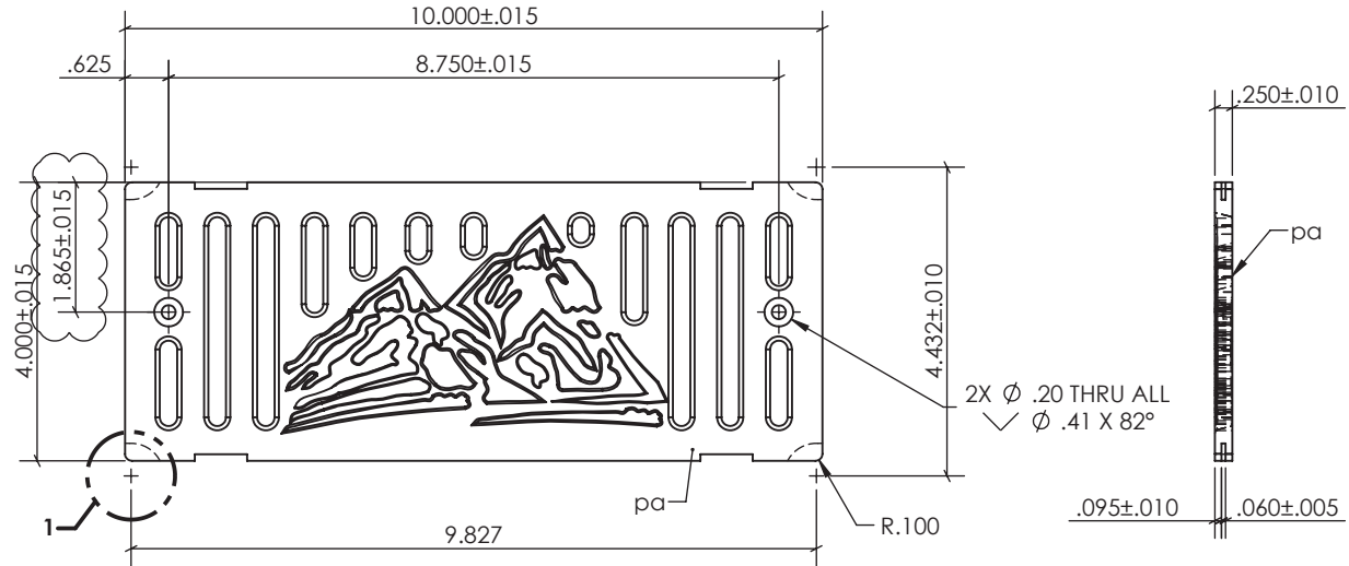
DETAIL: VI-4x10-A
